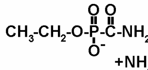
Fosamine ammonium salt
